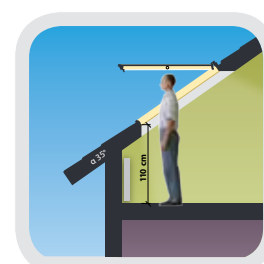
Klapp-Schwing-Fenster
